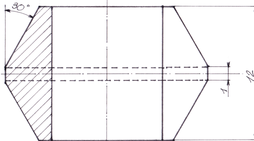
Coupe A-A
