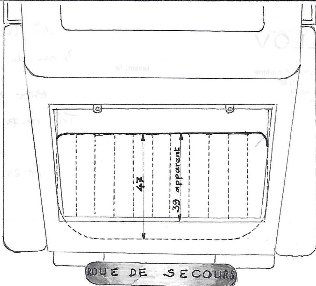
VUE DE DESSUS DU COFFRE OUVERT AVEC BANQUETTE EN PLACE
