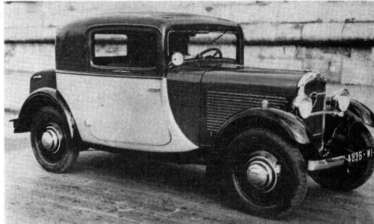
Le « coupé-décapotable de voyage » sur châssis « 201 C »
